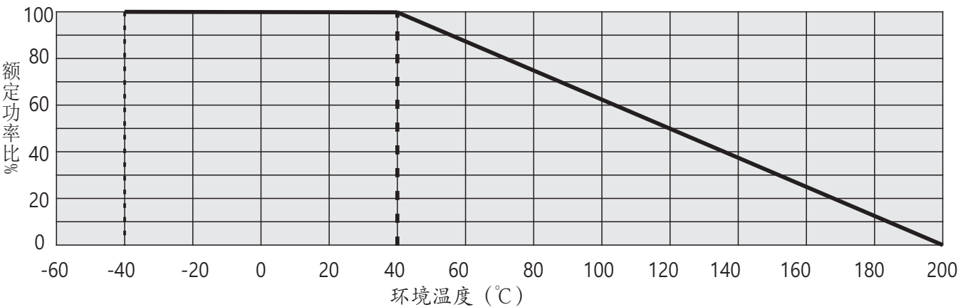
在环境温度70℃以上使用时，减小额定功率。
